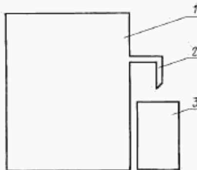
1 — сосуд; 2 — трубка; 3 — емкость для сбора воды
